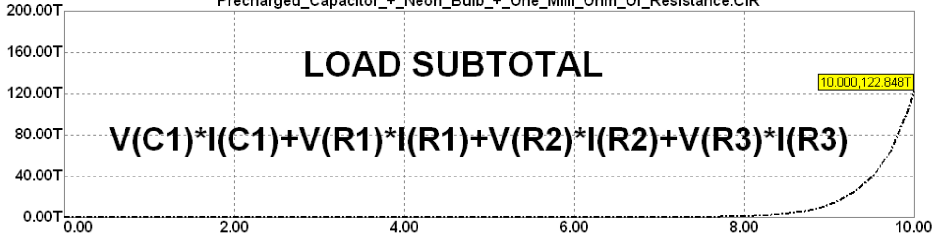
Precharged_Capacitor+_Neon_Bulb+_One_Milli_Ohm_Of_Resistance.CIR
