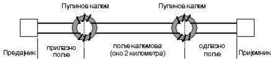
шема Пупиновог вода
